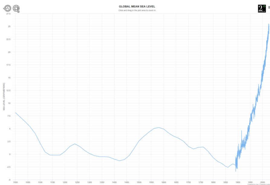
Figur 24 - Global havsnivå sedan år 1000
