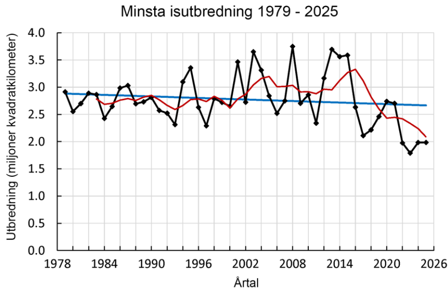
Figur 27 - Isutbredningen i Antarktis National Snow and Ice Data Center [25]
