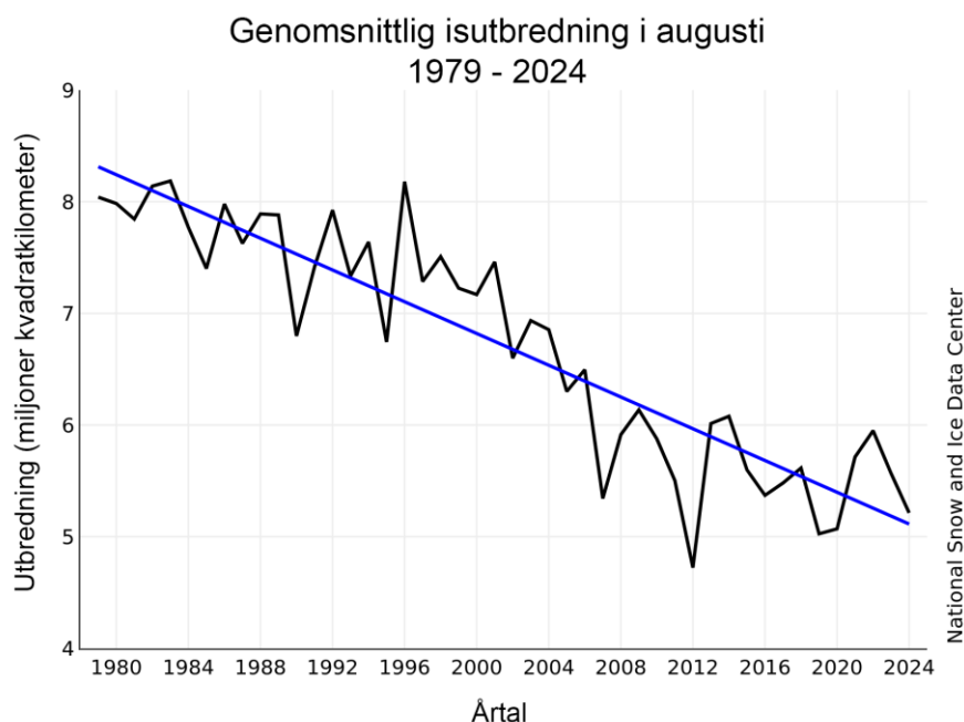
Figur 26 - Utbredning av sommarisen i Arktis National Snow and Ice Data Center [24]
