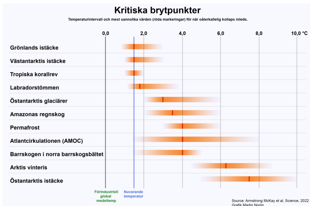
Figur 33. Kritiska brytpunkter Eget arbete baserat på data från Armstrong McKay et al. Science [26]
