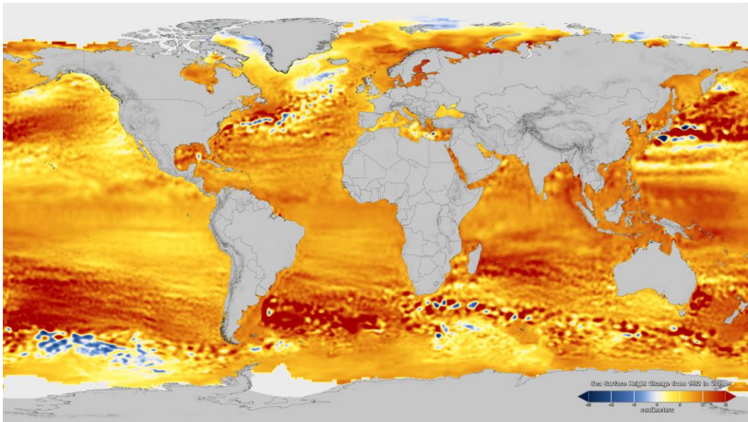
Figur 25 - Global havsnivåändring mellan 1993 och 2019 NASA [23]
